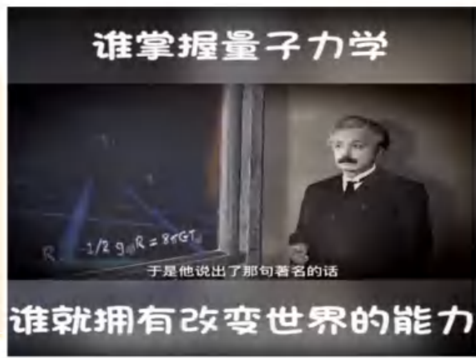
现代物理学两大支柱之一：量子力学
