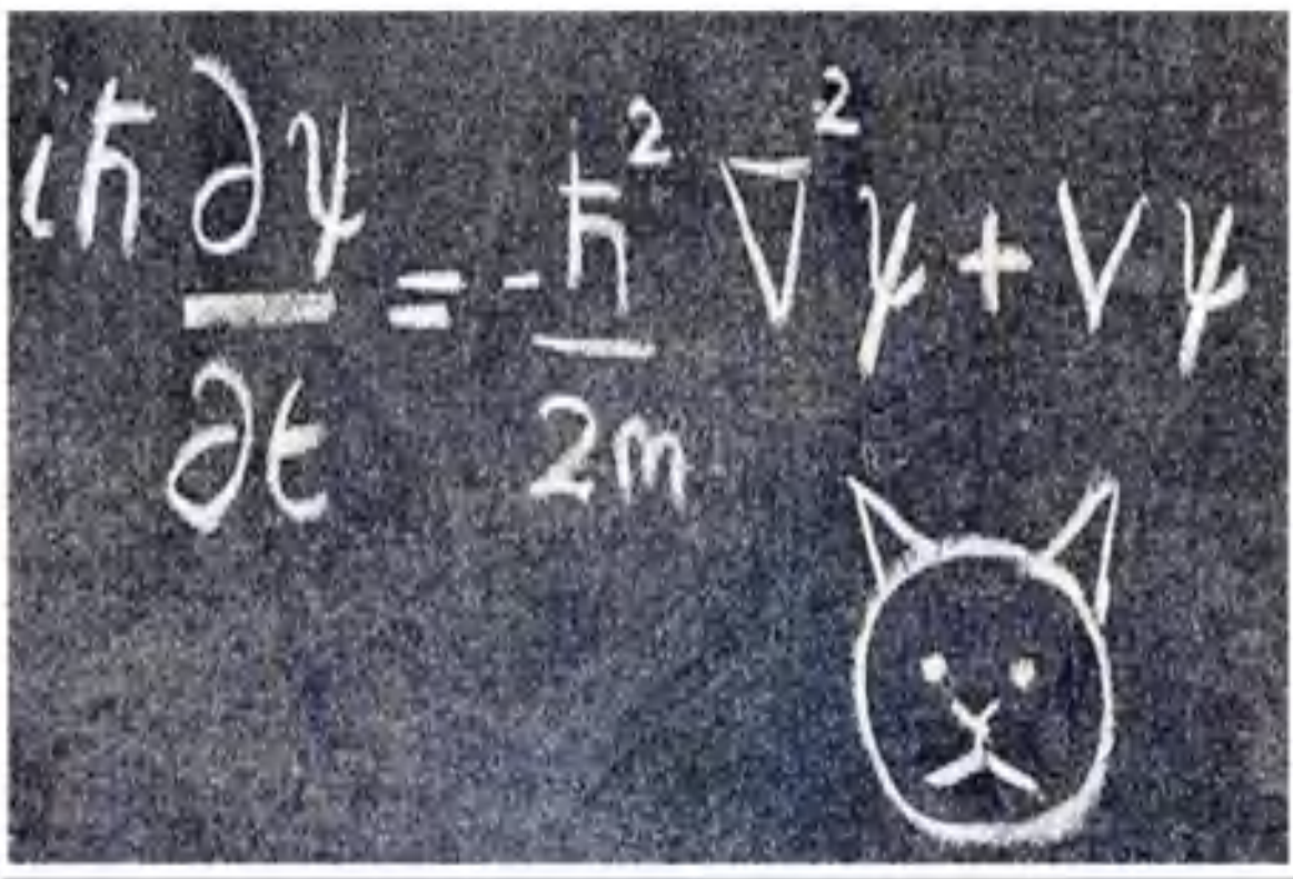
薛定谔方程是量子力学中的一个基本方程
