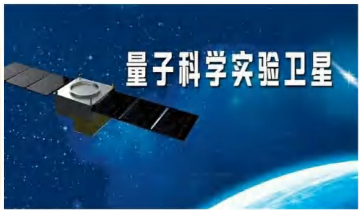
现代通信技术的新方向：量子通信
