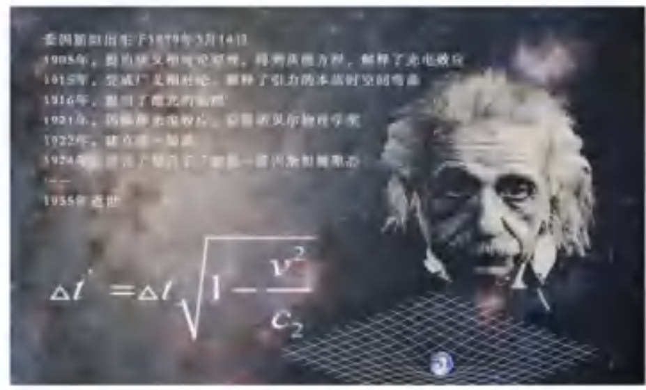
狭义相对论的钟慢尺缩效应
